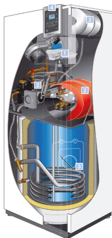
Effnox Condens Duo Version sol avec ballon intégré de 130L
